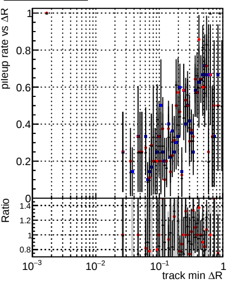
Legend: DQMstep3_DisplacedSUSY_CKF (blue), DQMstep3_DisplacedSUSY_default (red), DQMstep3_DisplacedSUSY_NEWT (black)
