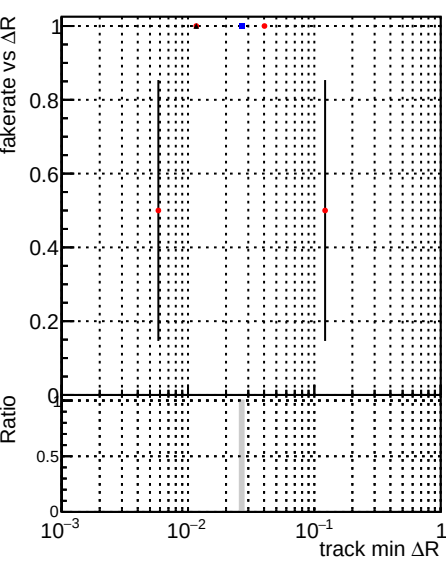
Fake rate vs \Delta R(\text{track, jet}) DQMstep3_DisplacedSUSY_CKF DQMstep3_DisplacedSUSY_default DQMstep3_DisplacedSUSY_defaultNEWT
