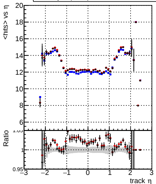
mean hits vs \eta — DQMstep3_DisplacedSUSY_CKF — DQMstep3_DisplacedSUSY_default — DQMstep3_DisplacedSUSY_defaultNEWT
