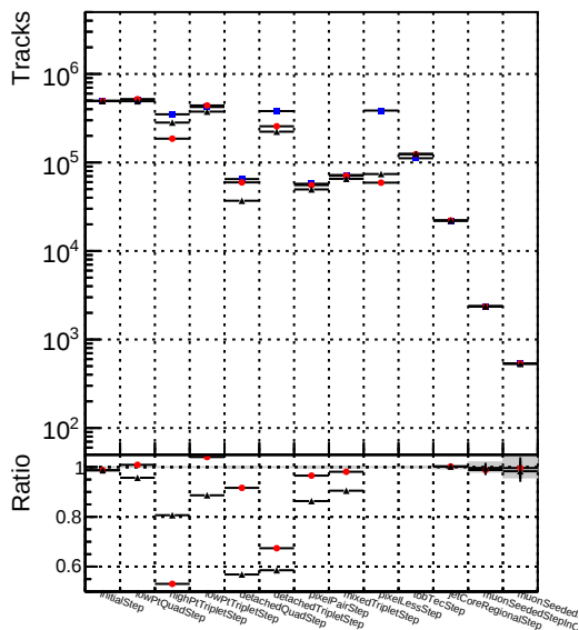
Number of tracks vs collection DQMstep3_DisplacedSUSY_CKF DQMstep3_DisplacedSUSY_default DQMstep3_DisplacedSUSY_defaultNEWWT
