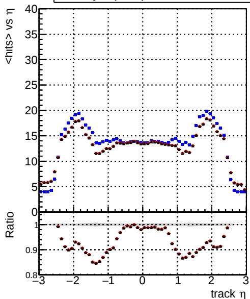
mean hits vs \eta DQMstep3_DisplacedSUSY_CKF DQMstep3_DisplacedSUSY_default DQMstep3_DisplacedSUSY_defaultNEWT
