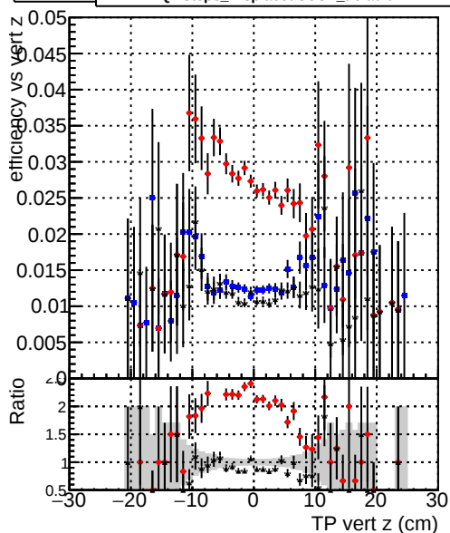
Efficiency vs vert z —●— DQMstep3_DisplacedSUSY_CKF —●— DQMstep3_DisplacedSUSY_default —●— DQMstep3_DisplacedSUSY_defaultNEWT
