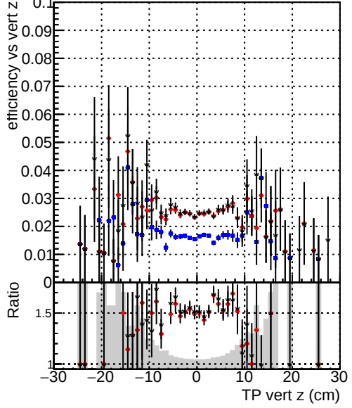
Efficiency vs. TP vert z (cm) — DQMstep3_DisplacedSUSY_CKF — DQMstep3_DisplacedSUSY_default — DQMstep3_DisplacedSUSY_defaultNEWT
