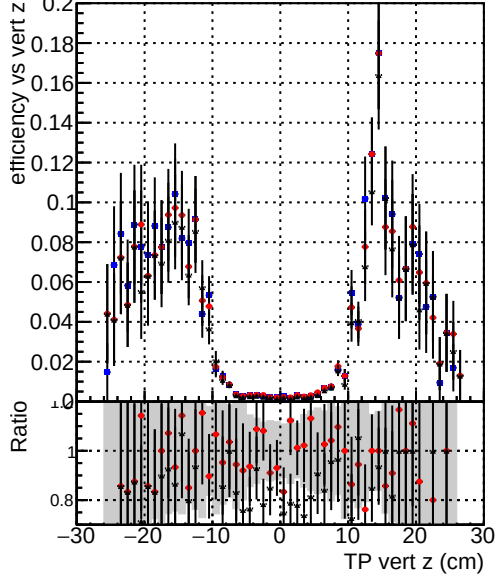
Efficiency vs. TP vert z —●— DQMstep3_DisplacedSUSY_CKF —●— DQMstep3_DisplacedSUSY_default —●— DQMstep3_DisplacedSUSY_defaultNEWT
