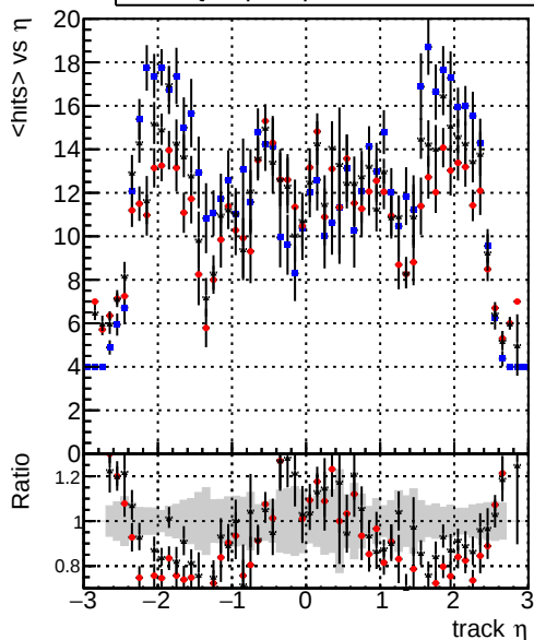
mean hits vs \eta — DQMstep3_DisplacedSUSY_CKF — DQMstep3_DisplacedSUSY_default — DQMstep3_DisplacedSUSY_defaultNEWT
