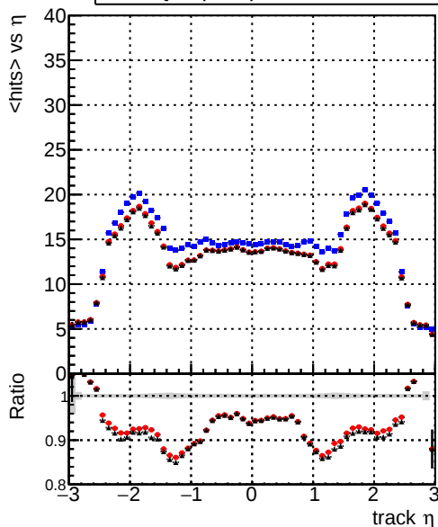
mean hit — DQMstep3_DisplacedSUSY_CKF — DQMstep3_DisplacedSUSY_default — DQMstep3_DisplacedSUSY_defaultNEWT
