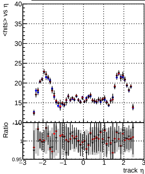
mean hits — DQMstep3_DisplacedSUSY_CKF — DQMstep3_DisplacedSUSY_default — DQMstep3_DisplacedSUSY_defaultNEWT
