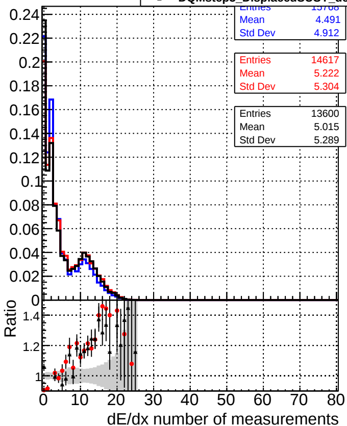
—■— DQMstep3_DisplacedSUSY_CKF —●— DQMstep3_DisplacedSUSY_default —*— DQMstep3_DisplacedSUSY_defaultNEWT
