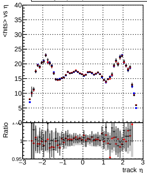
mean hits — DQMstep3_DisplacedSUSY_CKF — DQMstep3_DisplacedSUSY_default — DQMstep3_DisplacedSUSY_defaultNEWT
