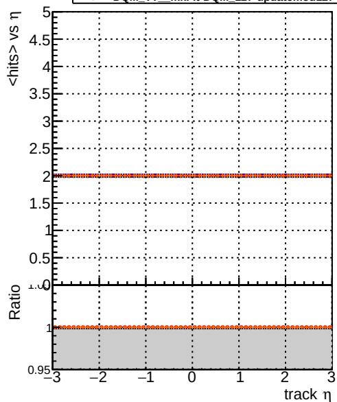
mean hits — DQM TT mkFit-DQM original — /data2/legianni/standalone-May24/CMSSW_13_2_X_2023-06-05-1100/src/DQM TT_mkFit-DQM_mod updatedmod127 — DQM TT mkFit-DQM_update-mod127 — DQM TT mkFit-DQM_127-updatemod127
