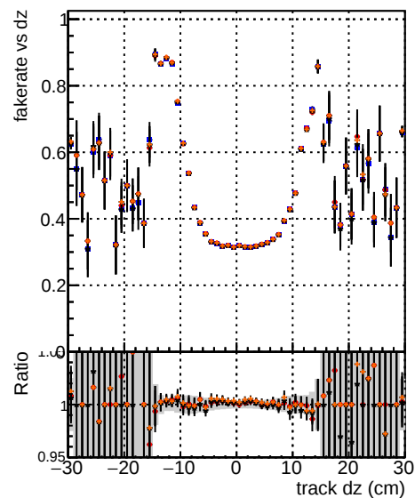
DQM TT mkFit-DQM_mod_updatedmod127 DQM TT mkFit-DQM_mod_updatedmod127 DQM TT mkFit-DQM_mod_updatedmod127
