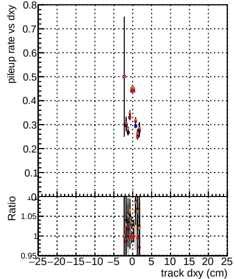
DQM_mod_updatedmod
