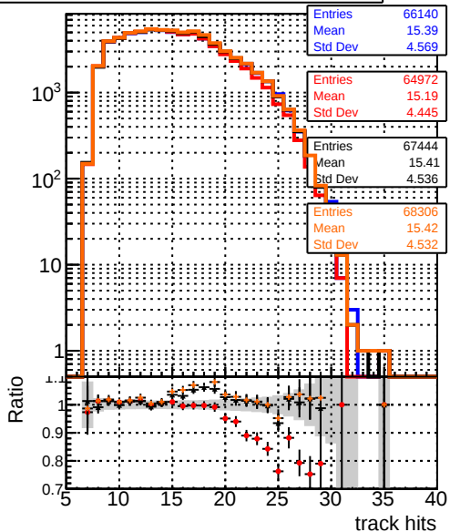
— DQM TT mkFit-DQM original — /data2/legianni/standalone-May24/CMSSW_13_2_X_X-2023-06-05-1100/src/DQM TT_mkFit-DQM_mod_updatedmod127 — DQM TT mkFit-DQM_update-mod127 — DQM TT mkFit-DQM_127-updatemod127
