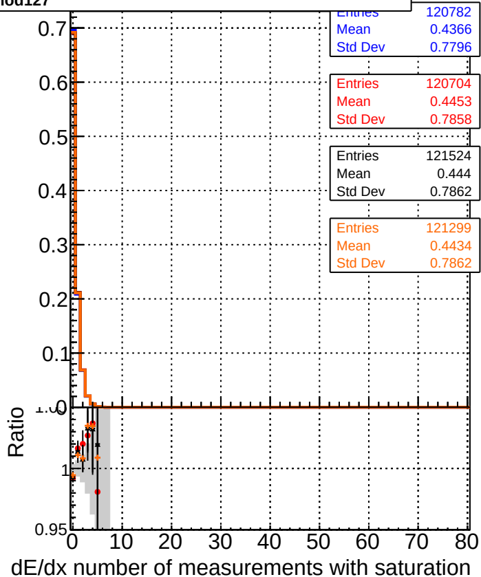
— DQM TT mkFit-DQM_original — /data2/legianni/standalone-May24/CMSSW_13_2_X_2023-06-05-1100/src/DQM TT mkFit-DQM_mod_upd — DQM TT mkFit-DQM_update-mod127 — DQM TT mkFit-DQM_127-updatemod127
