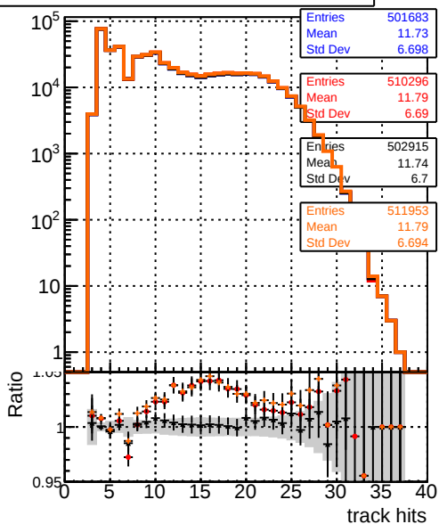
— DQM TT mkFit-DQM original — /data2/legianni/standalone-May24/CMSSW_13_2_X_X-2023-06-05-1100/src/DQM TT_mkFit-DQM_mod_updatedmod-127 — DQM TT mkFit-DQM_update-mod127 — DQM TT mkFit-DQM_127-updatemod127
