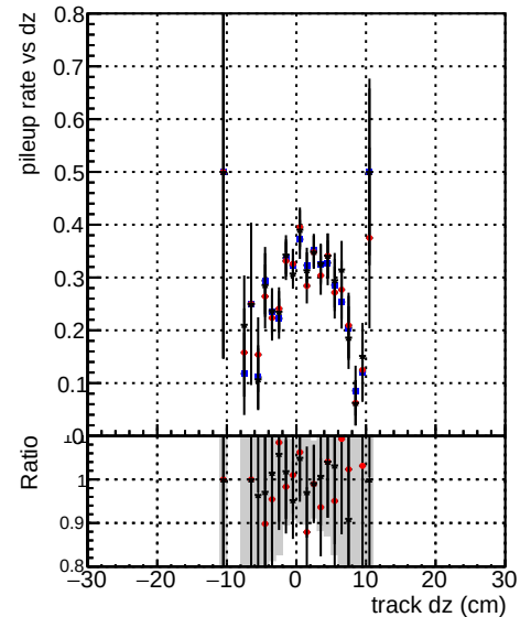
DQM_mod_updatedmo
