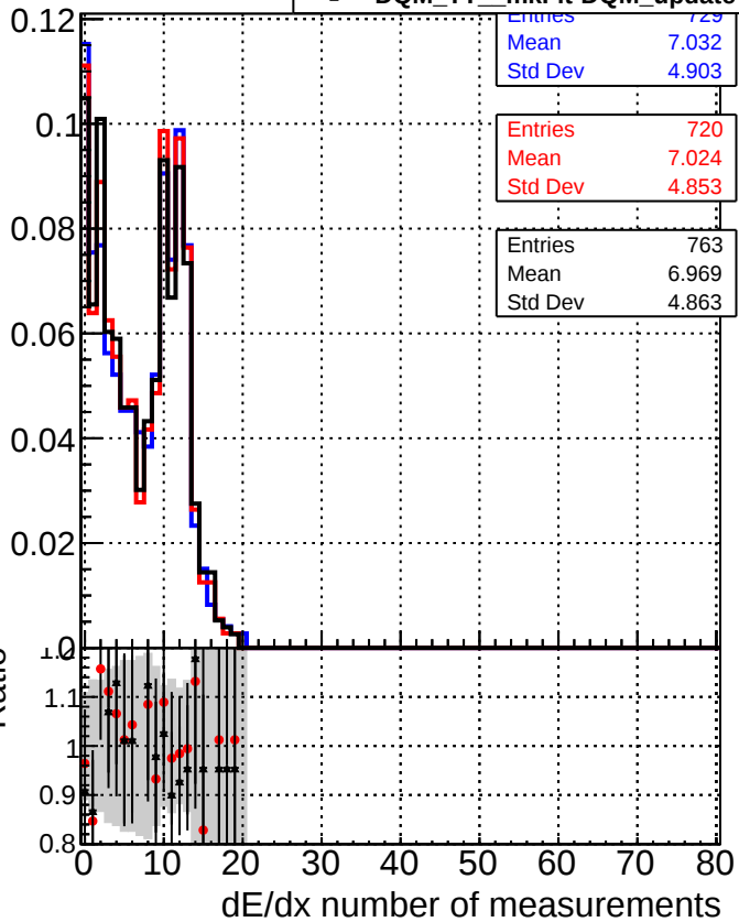
DQM_TT_mkFit-DQM_update-mod127
