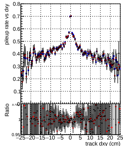
—•— DQM TT mkFit-DQM original —•— DQM TT mkFit-DQM update-mod127 —•— DQM TT mkFit-DQM update-mod127
