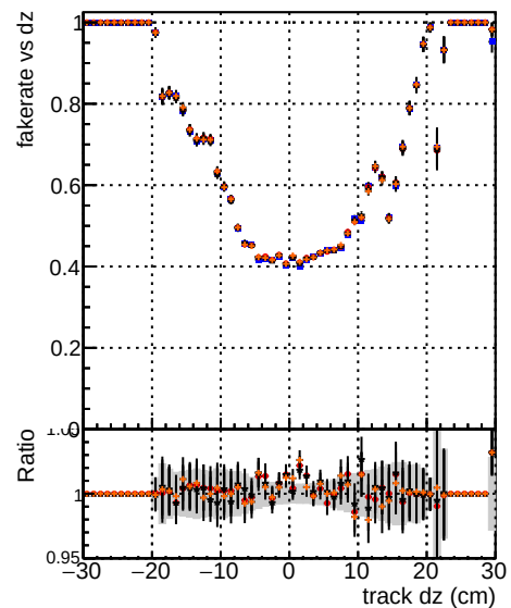
DQM TT mkFit-DQM-original DQM TT mkFit-DQM-updated-0 DQM TT mkFit-DQM-updated-mod127
