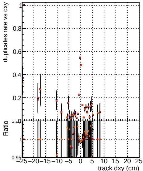
DQM TT mkFit-DQM-original DQM TT mkFit-DQM-updated-0 DQM TT mkFit-DQM-updated-mod127
