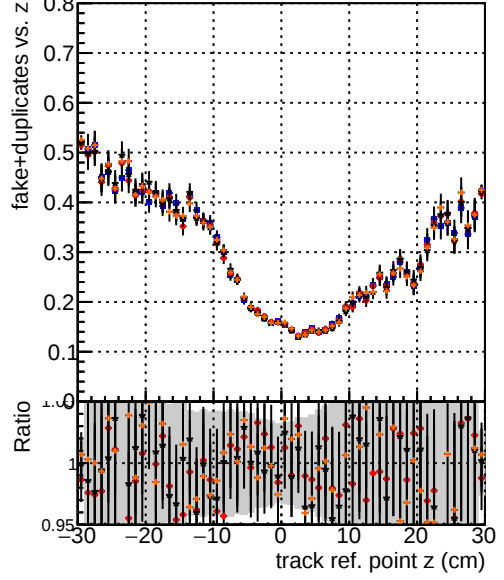
—●— DQM TT mkFit-DQM original —●— /data2/legianni/standalone-May24/CMSSW_13_2_X_2023-06-05-1100/src/DQM TT mkFit-DQM_updated0 —●— DQM TT mkFit-DQM original_newwindows —●— DQM TT mkFit-DQM update-mod127
