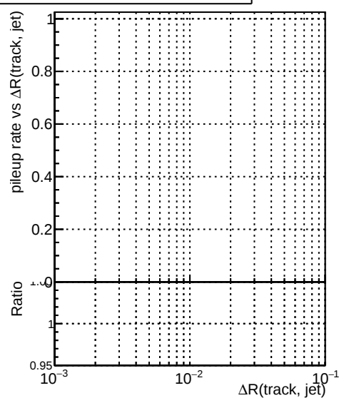
DQM_11_mkFit-DQM_updated-0
