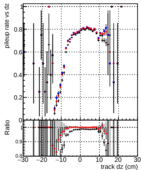
DQM_updated-0
