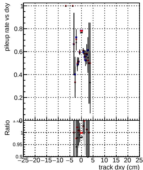
DQM_updated-0
