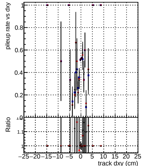
-DQM_updated-0
