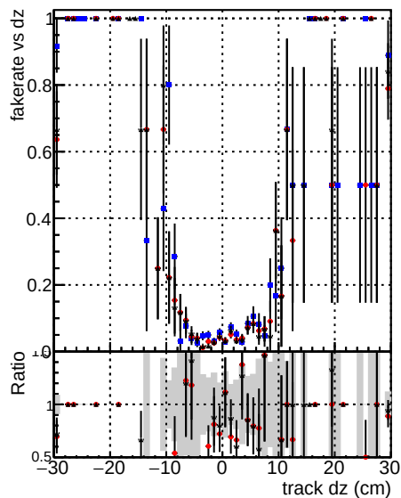
Legend: DOM CKF TTbar PU Fake rate vs d — DOM CKF TTbar PU — noDNN-baseline Duplicates rate vs d — DOM CKF TTbar PU — noDNN-fix
