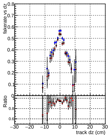
— DOM CKF TTbarPU — DOM CKF TTbarPU-noBNN-fix — DOM mktT TTbarPU-noBNN-fix
