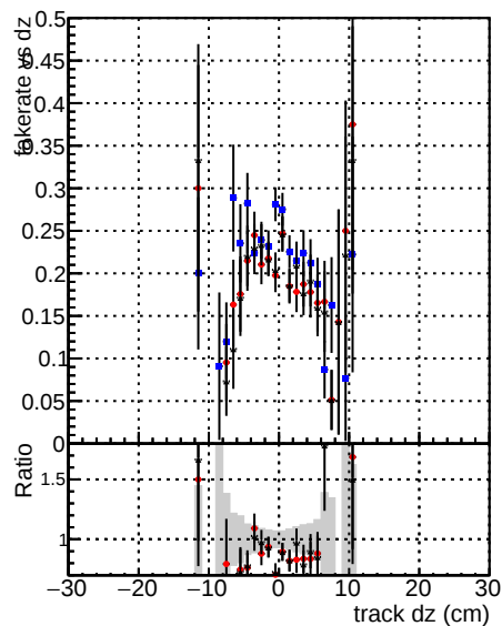
—•— DOM CKF TTbar PU —•— DOM CKF TTbar PU noBNN-baseline
