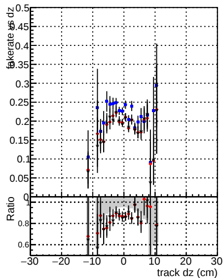
— DOM CKE TTbarPU — DOM mktFit TTbarPU-noBNN-fix
