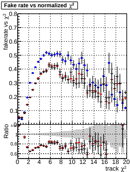
Fake rate vs. DOM CKF TTbar PU DOM mkt TTbar PU noBNN-baseline
