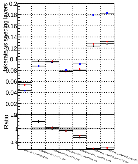
Fake rate vs. DOM CKF TTbar PU DOM mkt TTbar PU noBNN-baseline
