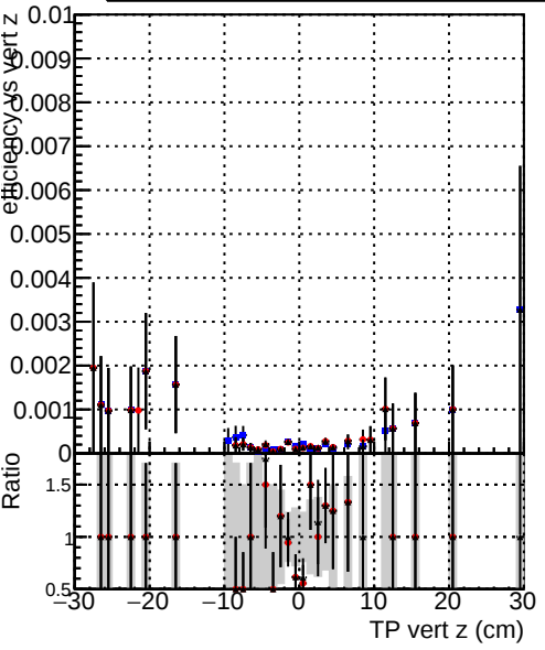
Efficiency vs TP vert z (cm) DQM_CKF_SoftQCD DQM_mkFit_SoftQCD-noDNN-baseline DQM_mkFit_SoftQCD-noDNN-fix
