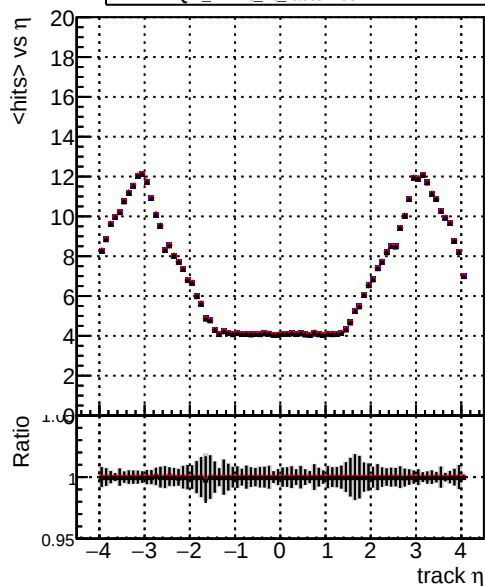
mean hits — DQM_mkFit_build — DQM_mkFit_fit — DQM_mkFit_fit_factor100
