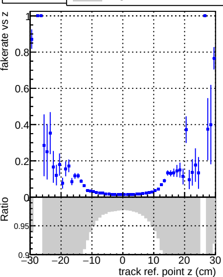
Fake rate vs v —■— DQM_TTPU_mkFit_BuildNewBaseline
