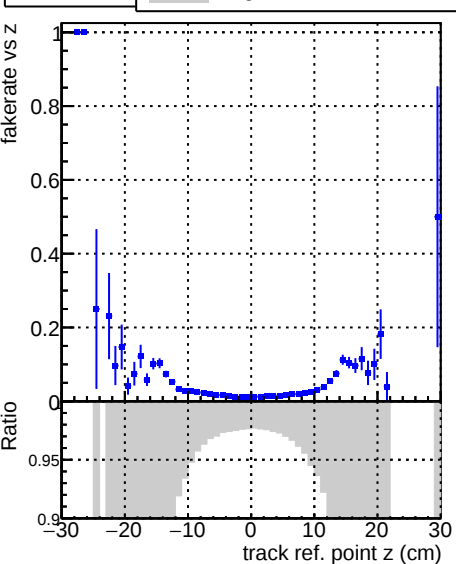
Fake rate vs vertpos DQM_TTPU_mkFit_BuildNewBaseline
