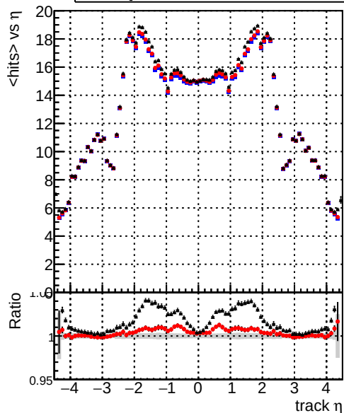
DQM_TTPU_mkFit_build DQM_TTPU_mkFit_Fit DQM_TTPU_mkFit_100RescaleBoth mean hits
