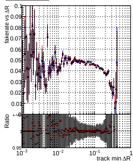
— DQM_TTPU_mkFit_BuildNEW2 — DQM_TTPU_mkFit_FitNEW2 — DQM_TTPU_mkFit_NoFitNEW2
