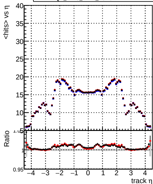
DQM_TTPU_mkFit_BuildNEW2 DQM_TTPU_mkFit_FitNEW2 DQM_TTPU_mkFit_NoFitNEW2 mean hits
