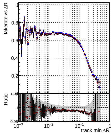
—•— DQM_TTPU_mkFit_BuildNEW2 —•— DQM_TTPU_mkFit_FitNEW2 —•— DQM_TTPU_mkFit_FitNEW3
