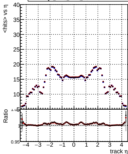
mean hits vs \eta — DQM_TTPU_mkFit_BuildNEW2 — DQM_TTPU_mkFit_FitNEW2 — DQM_TTPU_mkFit_FitNEW3
