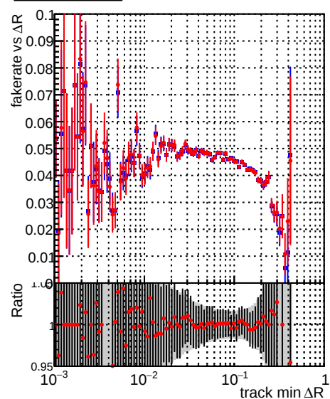
—•— DQM_TTPU_mkFit_BuildNEW2 —•— DQM_TTPU_mkFit_FitNEW2
