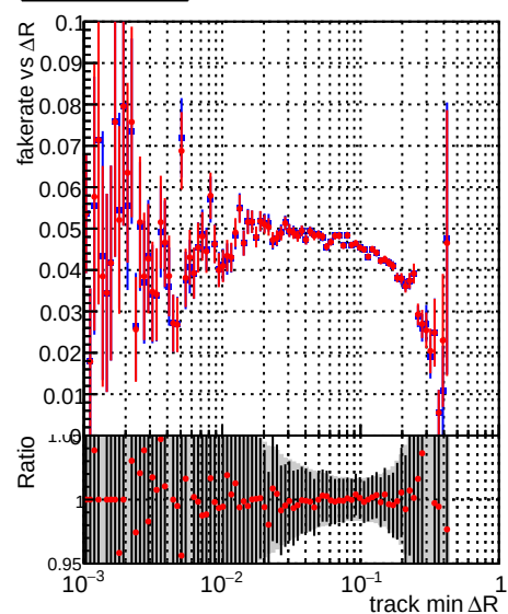
—•— DQM_TTPU_mkFit_build —•— DQM_TTPU_mkFit_BuildNEW
