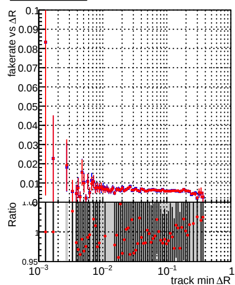
—•— DQM_TTPU_mkFit_BuildREDO_nofix —•— DQM_TTPU_mkFit_BuildREDO
