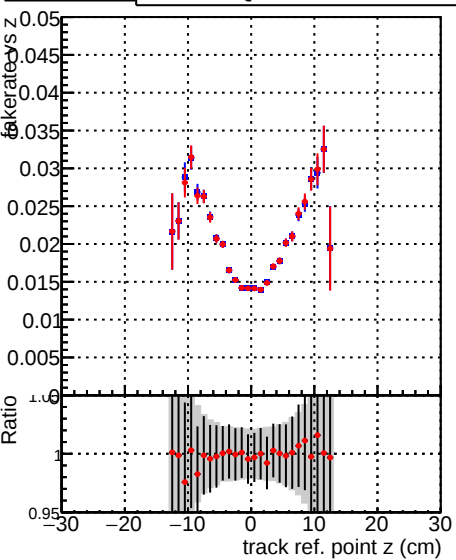
—●— DQM_TTPU_mkFit_BuildNewBaseline —●— DQM_TTPU_mkFit_BuildNewBaseline2
