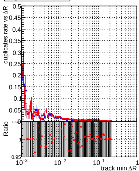
—•— DQM_TTPU_mkFit_BuildNewBaseline —•— DQM_TTPU_mkFit_BuildNewBaseline2
