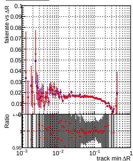
—•— DQM_TTPU_mkFit_BuildNewBaseline —•— DQM_TTPU_mkFit_BuildNewBaseline2
