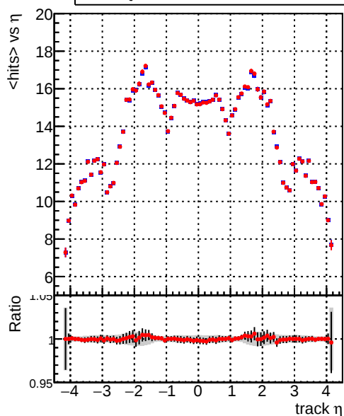
— DQM_TTPU_mkFit_FitNEW3 — DQM_TTPU_mkFit_FitNEW4 mean hits
