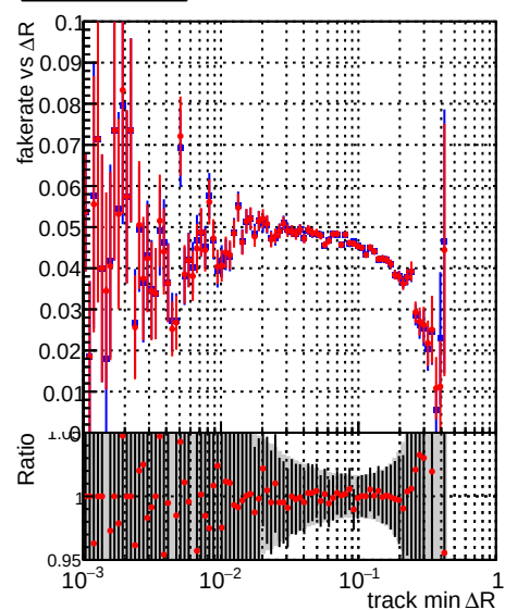
—•— DQM_TTPU_mkFit_BuildNEW4 —•— DQM_TTPU_mkFit_FitNEW4
