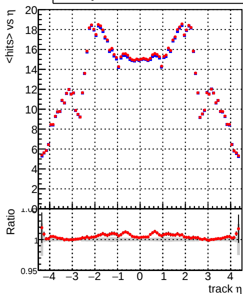
— DQM_TTPU_mkFit_BuildNEW4 — DQM_TTPU_mkFit_FitNEW4
