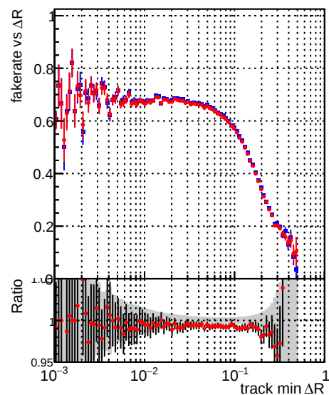
—•— DQM_TTPU_mkFit_BuildNEW4 —•— DQM_TTPU_mkFit_FitNEW4
